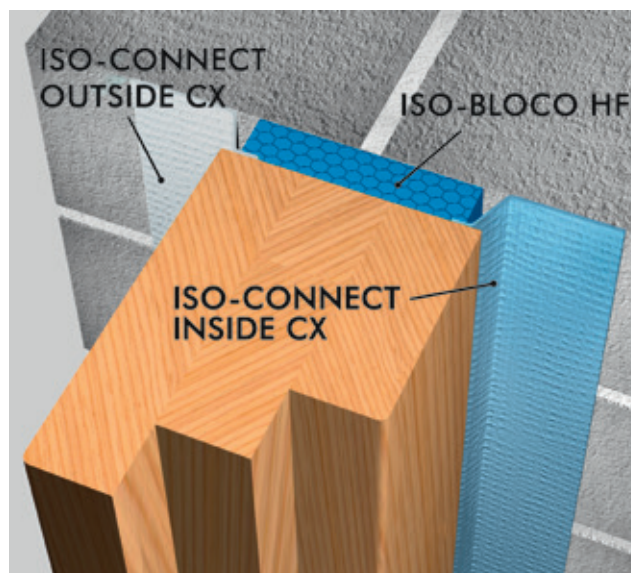
Einbaubeispiel: ISO³-FENSTERDICHTSYSTEM
